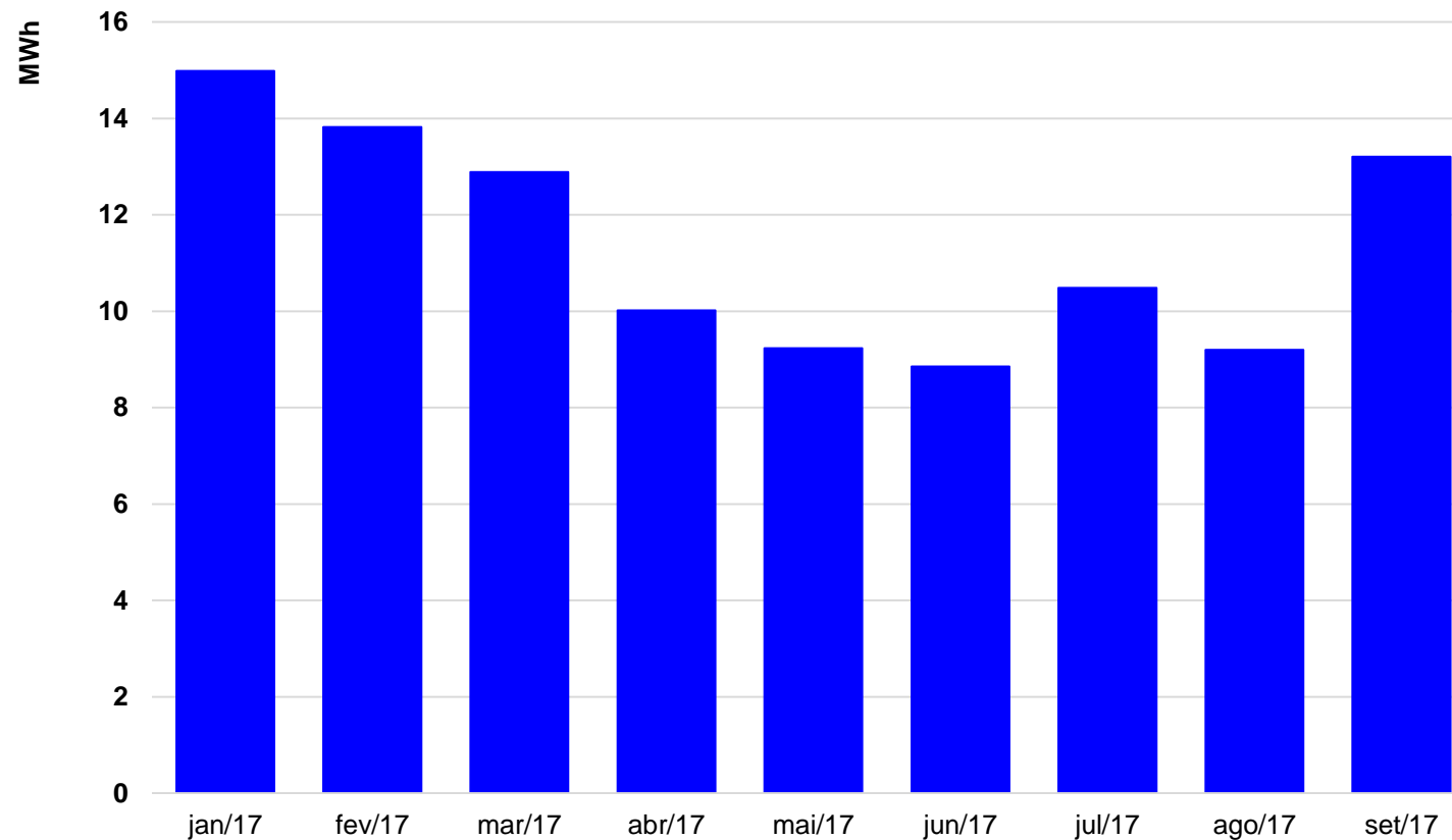
Figura 1. Geração de energia do sistema fotovoltaico.
