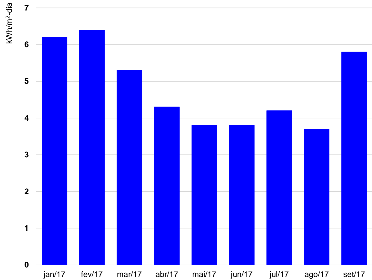
Figura 3. Radiação incidente nos módulos fotovoltaicos.
