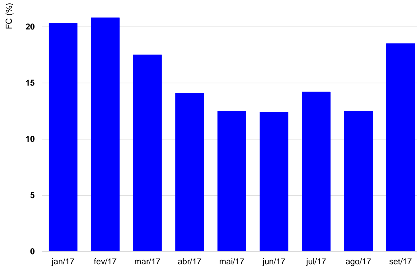
Figura 5. Fator de capacidade do sistema fotovoltaico.
